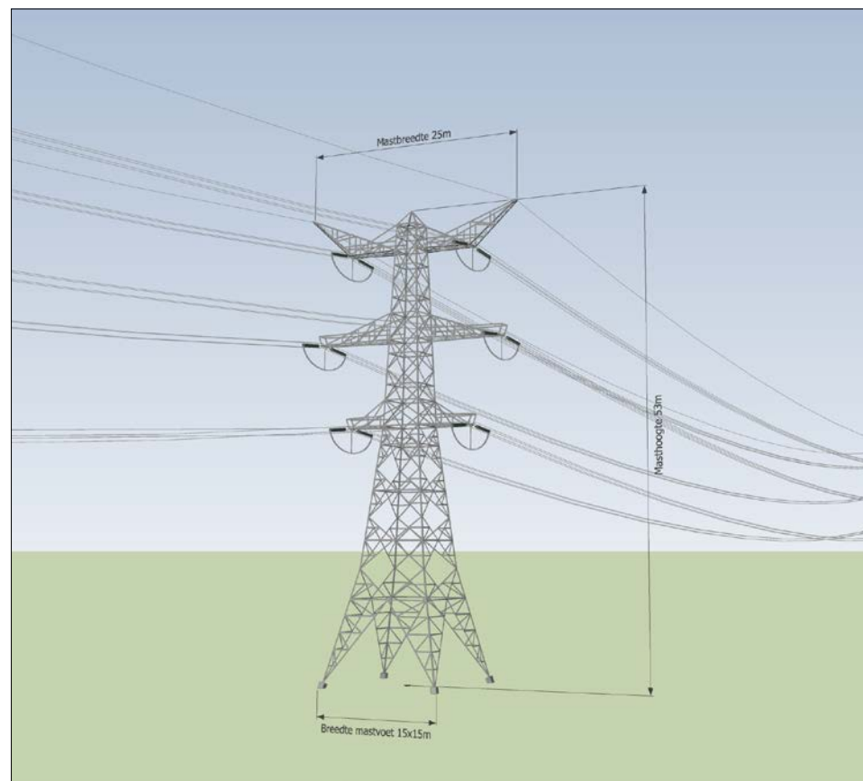
afb. 10 Moldau solomast 380kV - Trek/hoekmast
